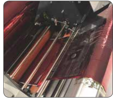
Hinteransicht der Matrix, die die Folienausgabe und -Aufnahme anzeigt
